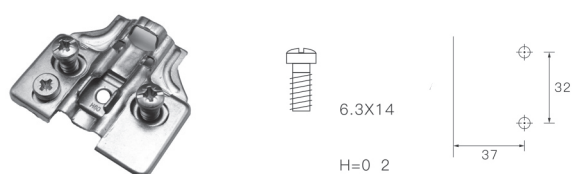
Монтажная планка с эксцентриковой регулировкой под евровинт
