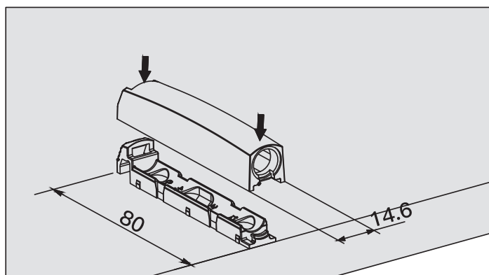
Накладной толкатель
