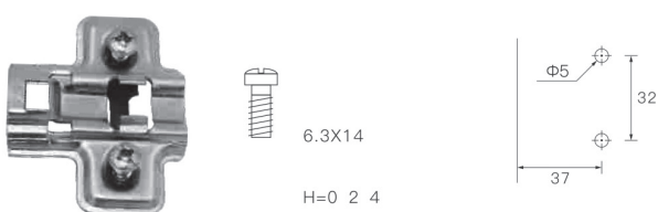
Монтажная планка с евровинтом
