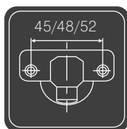
Межосевое расстояние
